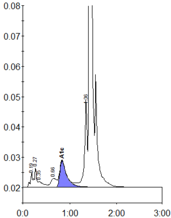
Peak table - ID: 10666726
